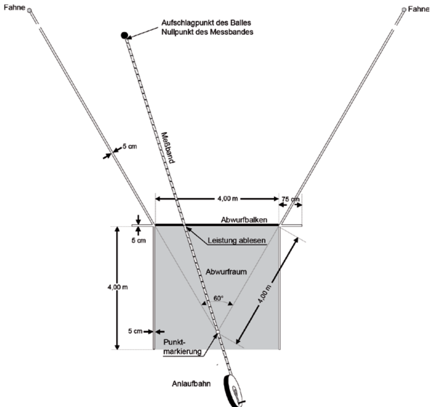
Maße zum Anlegen der Sektorlinien
